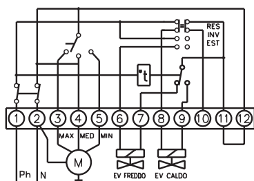
FT40
